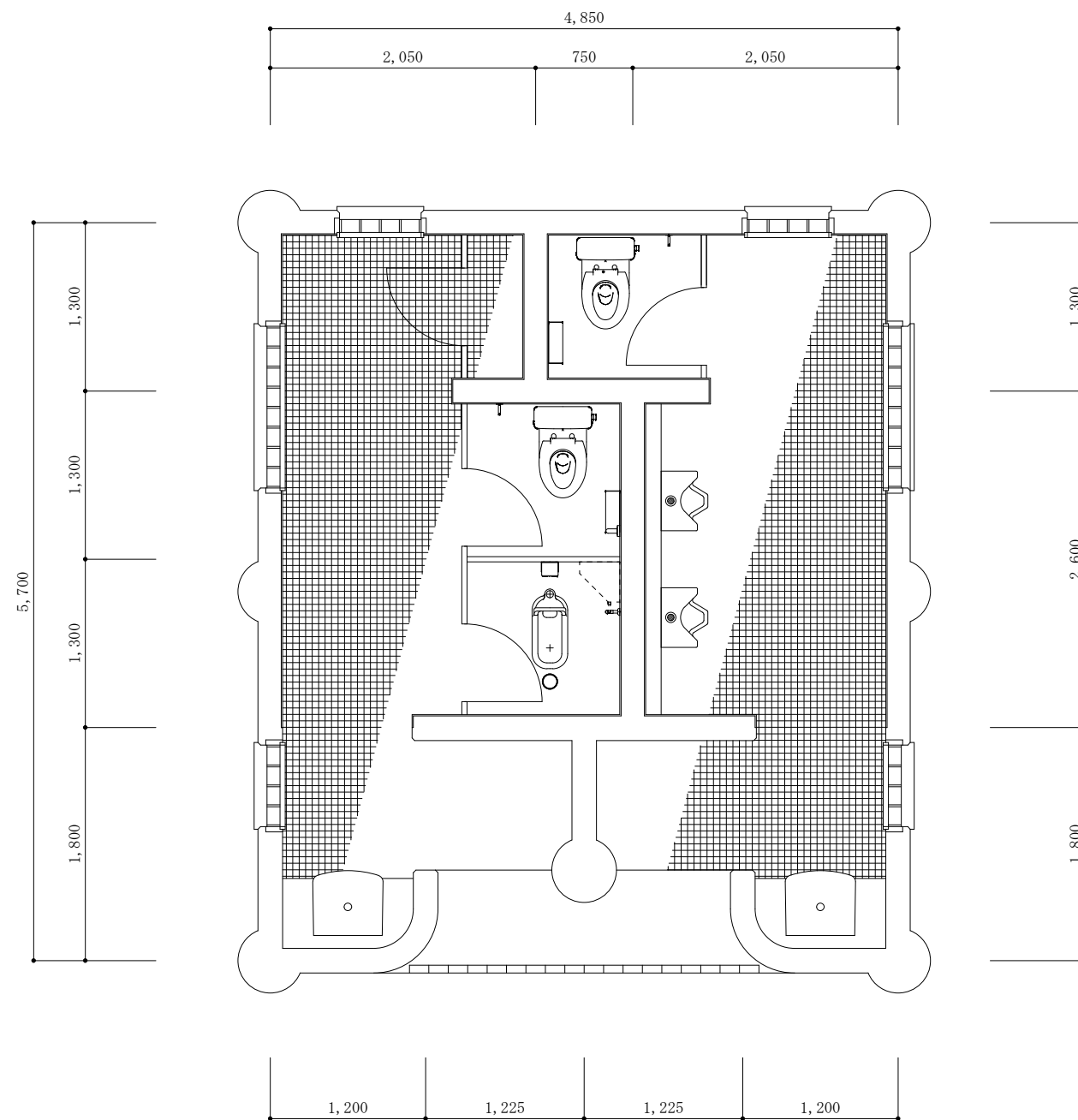
<平面図 1/50>
