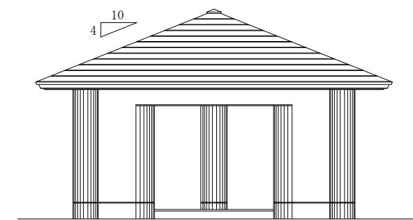
<南立面図 1/100>
