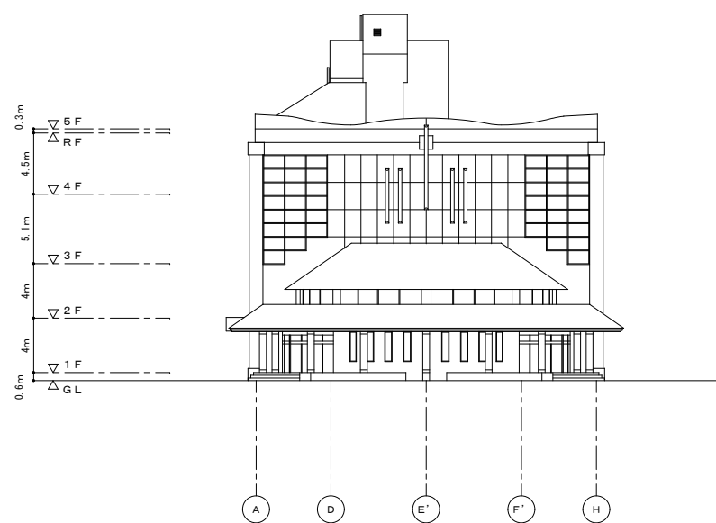
南 立面図 1:500
