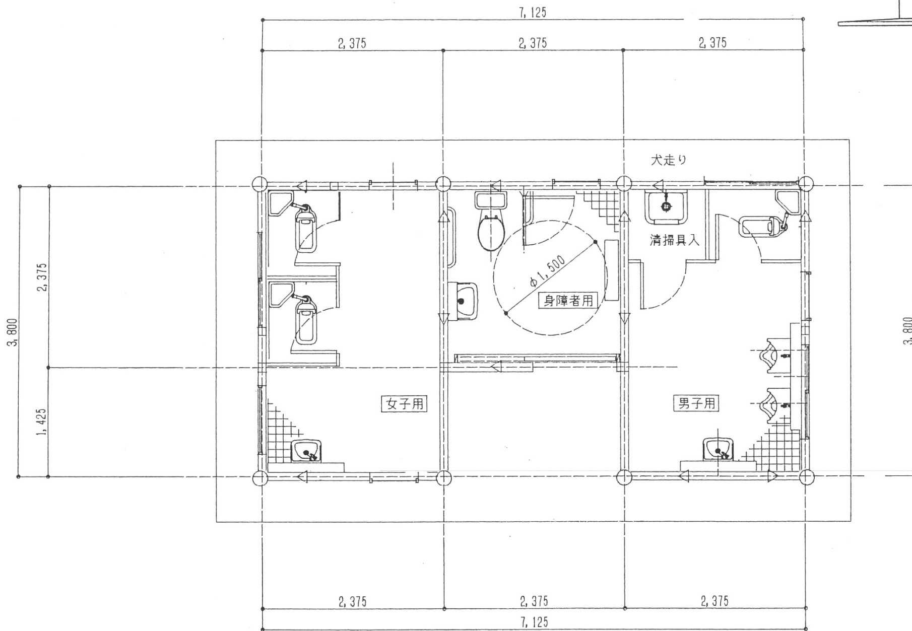
平面図 S=1/50
